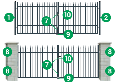
ZAUNFELD (Ansicht von der Straße)
