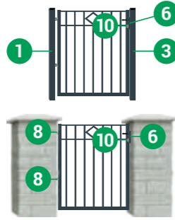
GARTENTOR LINKS* (Ansicht von der Straße)
