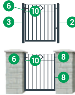
GARTENTOR RECHTS* (Ansicht von der Straße)
